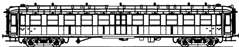
No cat. HO-120/1 PLM voiture C 11 "Bacalan", vert PLM, toit gris, bouts noirs No cat. HO-121/1 SNCF voiture C 11 "Bacalan" 1950, vert SNCF, toit et bouts noirs
