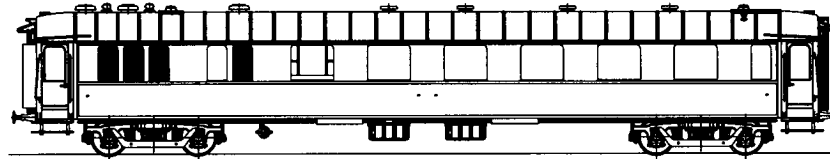
OCEM FL A 2 syfi "Transat", vert 2 tons, toit blanc
