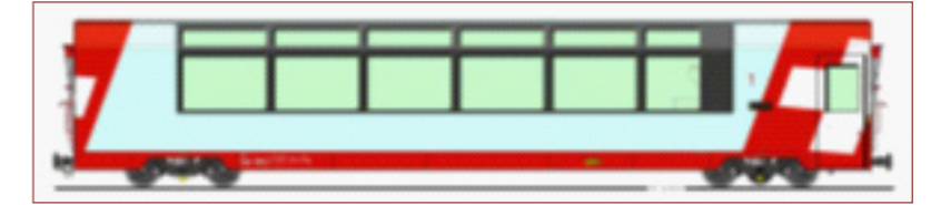
Aps «Excellence Class» Om-206/ 7A RhB Aps 1321 EC Om-206/ 7B MGB Aps 4046 EC
